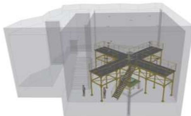
Systém kalibračních lavic pro neutronovou ozařovnu
